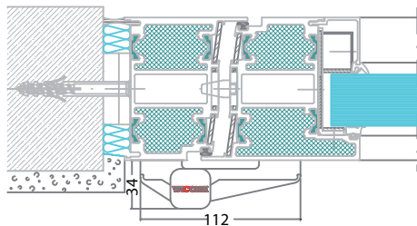
Frontmonterat gångjärn WICSTAR, aluminium
