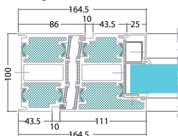
Dörrblad för smalprofilås
