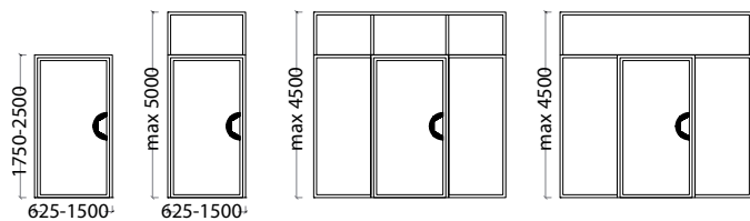
EI 90-1 dörr
