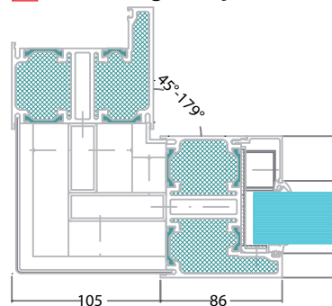
Hörn 90°
