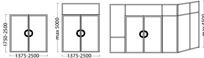
EI 90-2 pardörr
