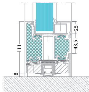
Tröskel mot golv
