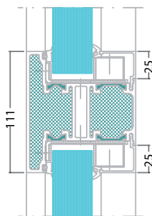
Spröjs
