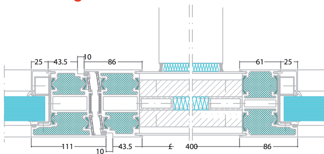
T-anlutning av innervägg
